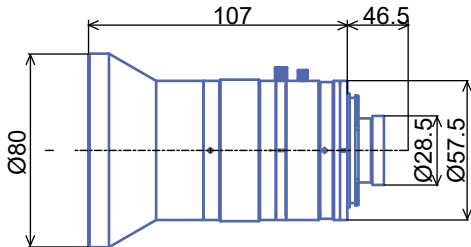
GLS8556M+ADP
