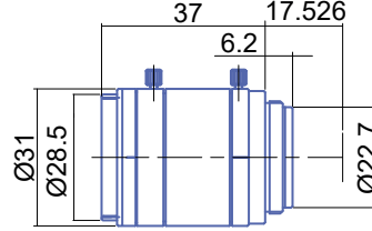
GMTHR33520MCN-1
