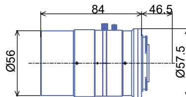
GLS5526F
