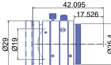
GMTHR33520MCN-1
