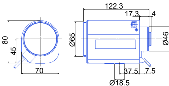
GAZMP30100M
