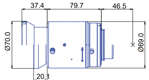
GM5HR612520MCN-SWIR
