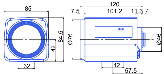
GAZMP31166M
