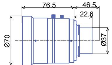
GLSW5028F
