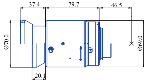
GLS5526F
