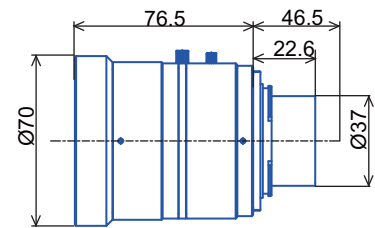
GLSW5028F
