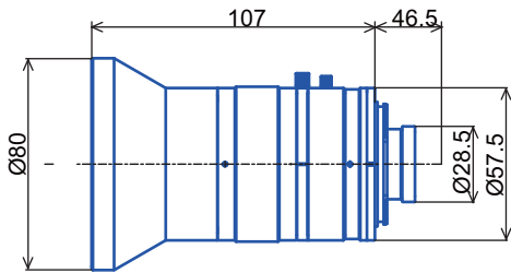
GLSW2528F
