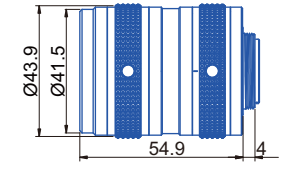
GM12HR38018MCN
