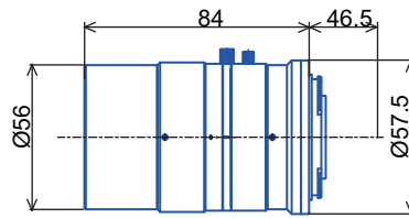
GLSW3528F
