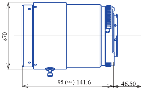
GLS10028F
