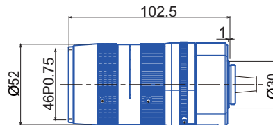
GMZ28585MCN
