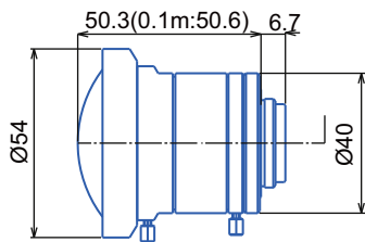
GMTHR46018MCN
